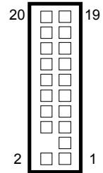
JLPC1
