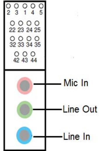
AUDIO1
