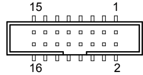
DIO1
