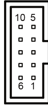
JAUDIO1
