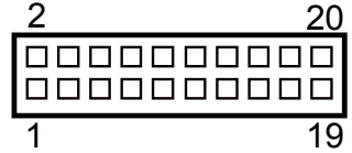
JDIO1
